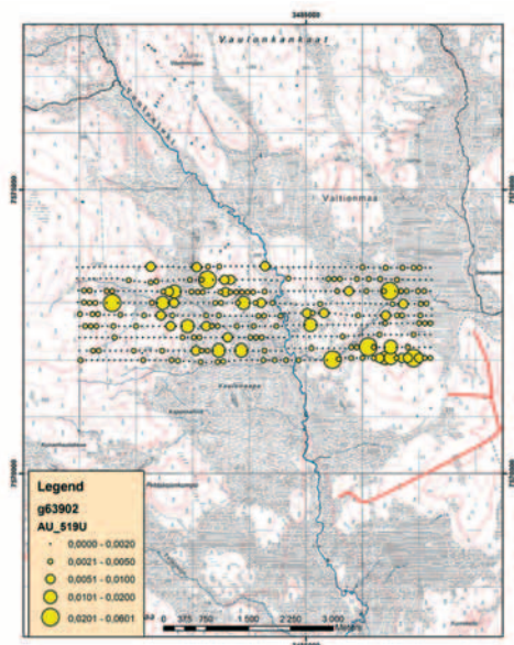
Kuva 2. Vaulojoen moreenin kulta-anomaliat ja sen itäpuoliseen aarreaittaan johtavien juontoteiden länsipäät. Kuva ei ulotu aivan Vaulon latvalle, missä Vaulon lammen kallio sijaitsee.
