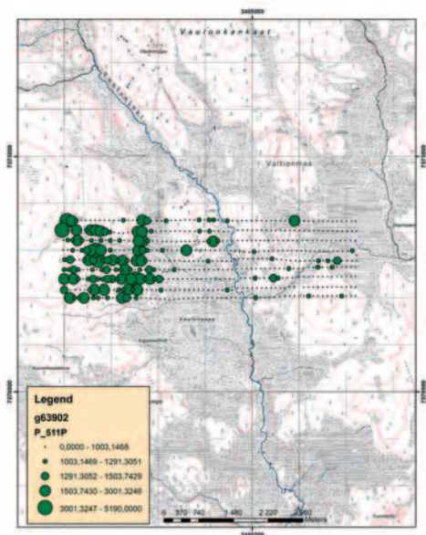
Kuva 4. Moreenin geokemian fosforipitoisuus (P) osoittaa Soklin malmintyyppistä esiintymää Vaulojoen länsipuolella.
