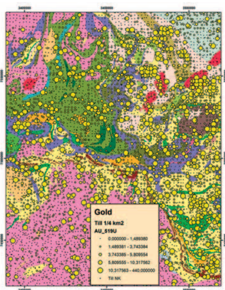
Kuva 1. Vaulojoen aarreaitta sijaitsee 40 kilometriä länteen valtatie 4:ltä ja sinne pääsee Vuotson ja Tanakavaaran väliltä länteen Mäkärröroville haarautuvaa soratietä pitkin. Oikeanpuolimmaisessa kuvassa on esitetty Keski-Lapin moreenin kultapitoisuudet.
