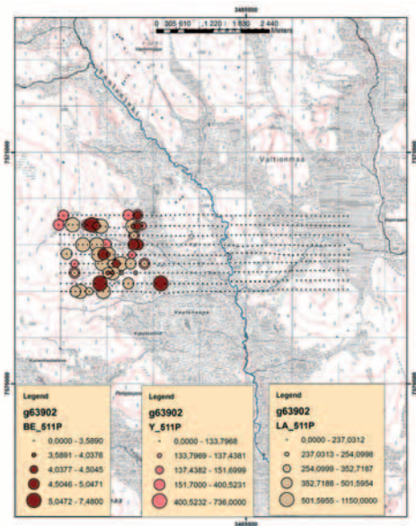
Kuva 3. Moreenin geokemian berylliumin (Be), yttriumin (Y) ja lantaanin (La) pitoisuudet osoittavat alkalikivimassiivin sijaintia.
