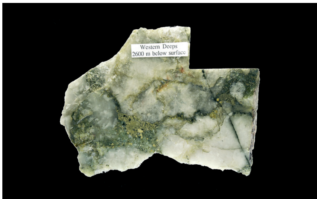
Witwatersrandin kultamalmia, joka on muinaista soraa, konglomeraattia. Valkoinen on kvartssia, kellertävä pyriittiä ja tumma kloriittia ja kiillettä. Malmikiven leveys on 12 cm. Näyte on GTK:n erikoistutkija Pasi Eilun kultamalmikokoelmasta. Kuva: Kari A. Kinnunen, GTK.
