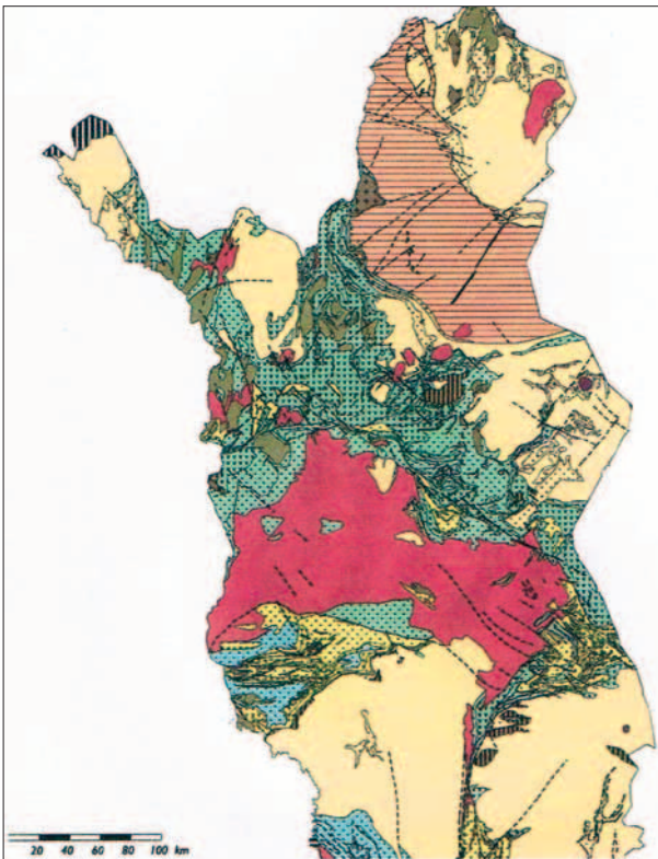
Kuva 4. Pohjois-Suomen kallioperä. Kartassa punainen symbolisoi graniittia, sininen ja keltainen sedimenteistä ja vulkaanista kivilajeista koostuvia pintakiviyksiköitä, vaaleanharmaa vastaa kaikkein vanhimpia arkeaisia kiviä, tummanruskeat ovat gabroa ja doleiriittia eli tummia syväkiviä kuten ruskealla pystyviivoitettu Koitelaisen gabro ja Käsivarressa on valkoisella pystyviivoitettu alue, joka on Kaledoniidien ylityöntölaatta. Suorat viivat osoittavat kallioperä heikkousvyöhykkeitä eli siirroksia. Silvennoinen, A., Gustavson, M., Perttunen, V., Siedlelecka, A., Sjöstrand, T. & Zachrisson, E. 1987. Geological map. Pre-Quaternary rocks. Northern Fennoscandia: Geological Surveys of Finland, Norway and Swedeninla.
