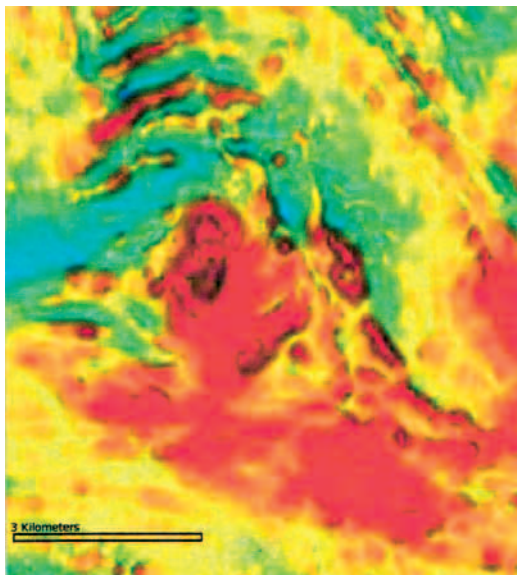
Kuva 5. Aeromagneettinen kartta. Mitä punaisempi, sitä enemmän on kallioperässä magnetiittia. Jolmavaara on punainen piste kartan alalaidassa, ja se ympäristöineen on samaa tasoa kuin Kolarin alueen rauta-kupari-kulta malmit.
